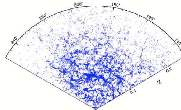
Galaxies
