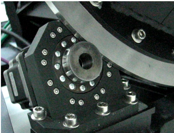
Przekładnia harmoniczna
