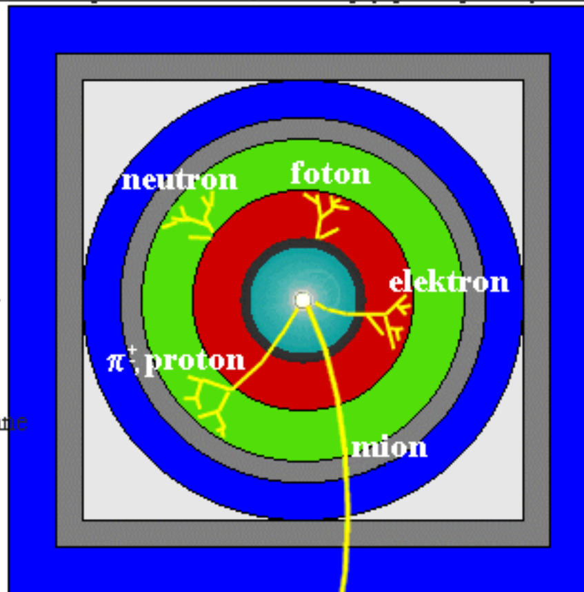
Przekrój poprzeczny detektora, ilustrujący torry cząstek
