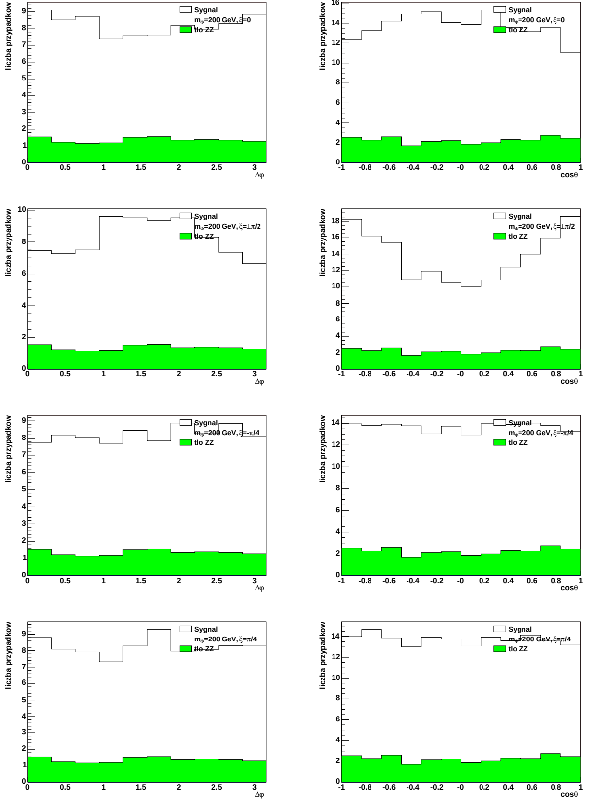
Rysunek 5.3: Zrekonstruowane po selekcji rozkłady kąta \varphi (rys. lewe) oraz cosinusa kąta \theta (rys. prawe) dla różnych wartości parametru \xi – patrząc od góry dla higgosa skalarnego, pseudoskalarnego oraz z \xi = -\pi/4, +\pi/4 . Histogramy niewypełnione odpowiadają sygnałowi o m_\phi = 200 GeV, zaś histogramy wypełnione tłu ZZ^* (pozostałe rodzaje tła są niewidoczne). Rysunki zostały znormalizowane do scałkowanej świetłości 20 \text{ fb}^{-1} .
