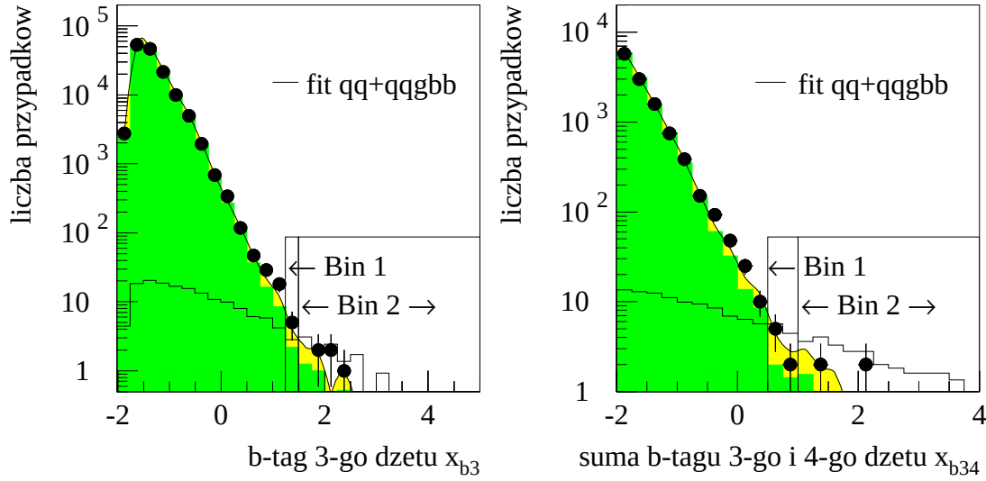
Rysunek 2.2: Rozkłady b-taggingu najsłabiej b-tagowanych dżetów. Punkty odpowiadają danym, ciemny histogram oczekiwanemu tłu (z g_{bb} = 1,5 \cdot 10^{-3} ), zaś histogram niewypełniony sygnałowi ( b\bar{b}(A \rightarrow b\bar{b}) , m_A = 40 GeV) znormalizowanemu arbitralnie. Dopasowanie oczekiwanego tła ( q\bar{q} + q\bar{q}(g \rightarrow b\bar{b}) ) do danych (jasny histogram) sugeruje większą wartość g_{bb} (zobacz rozdział 2.4.3).
