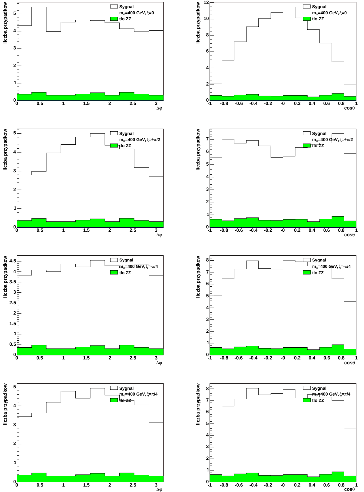
Rysunek 5.5: Zrekonstruowane po selekcji rozkłady kąta \varphi (rys. lewe) oraz cosinusa kąta \theta (rys. prawe) dla różnych wartości parametru \xi – patrząc od góry dla higgsa skalarnego, pseudoskalarnego oraz z \xi=-\pi/4, +\pi/4 . Histogramy niewypełnione odpowiadają sygnałowi o m_\phi=400 GeV, zaś histogramy wypełnione tłu ZZ^* (pozostałe rodzaje tła są niewidoczne). Rysunki zostały znormalizowane do skalkowanej światłości 20 \text{ fb}^{-1} .
