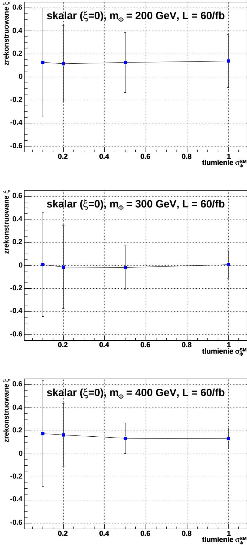
Rysunek 5.11: Zrekonstruowana wartość parametru \xi dla higgsa skalarnego w zależności od tłumienia przekroju czynnego sygnału w Modelu Standardowym ( \sigma_{\Phi}^{SM} ) dla mas (od góry) m_{\Phi}=200, 300, 400 GeV. Błędy odpowiadają jednemu odchyleniu standardowemu.
