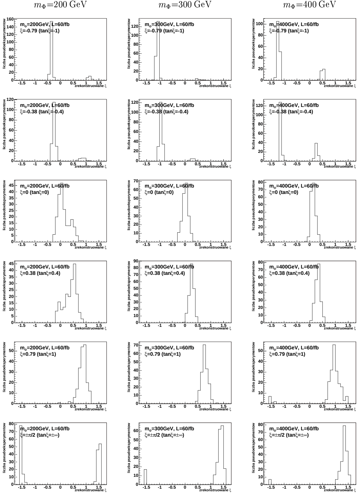
Rysunek 5.7: Rozkłady parametru \xi otrzymane dla 200 pseudoeksperymentów przy scałkowanej świetłości 60 \text{ fb}^{-1} . Kolejne kolumny (od lewej) odpowiadają masom higgsa m_\phi = 200, 300, 400 \text{ GeV} , zaś wiersze (od góry) odpowiednio \tan \xi = -1, -0.4 , skalarowi, \tan \xi = 0.4, 1 , pseudoskalarowi.
